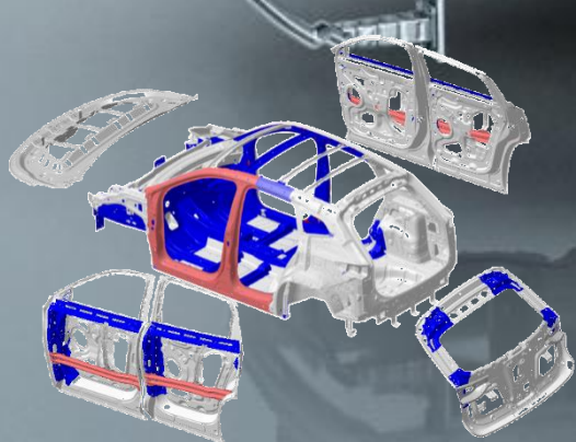
ساختار بدن از نوع قفس
